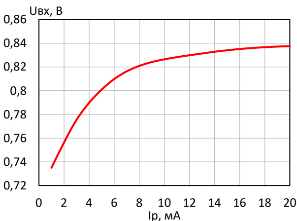
Входное напряжение покоя U вх при изменении режимного тока I p
