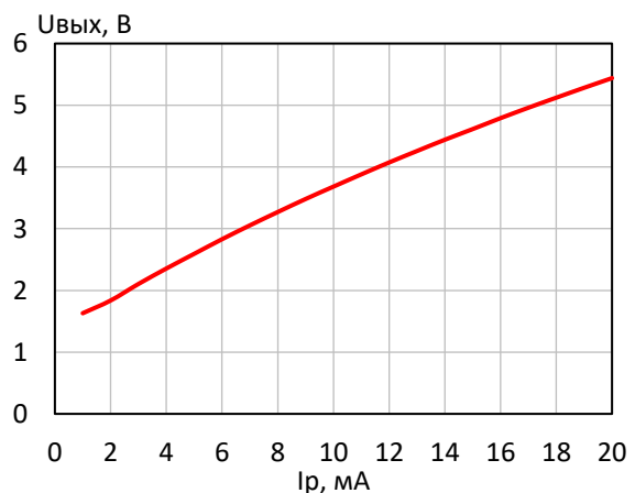
Выходное напряжение покоя U вых при изменении режимного тока I p
