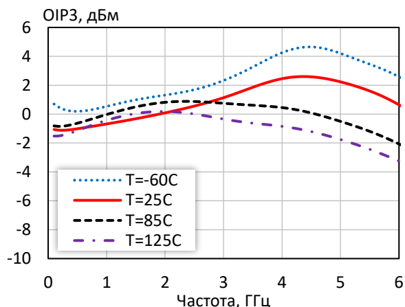
Точка пересечения интермодуляции третьего порядка по выходу при различной температуре ( I_p = 8\text{mA} )
