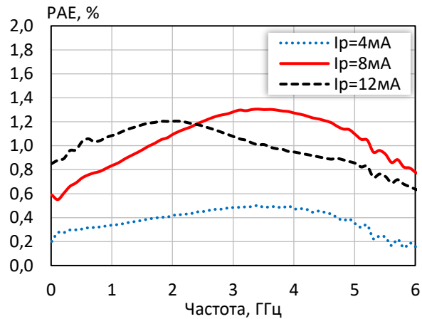
КПД по добавленной мощности в точке P вых3дБ при различных режимных токах
