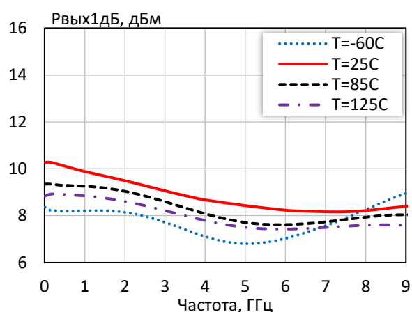
Выходная мощность при уровне компрессии K_{ур} на 1 дБ при различной температуре ( I_p = 30\text{ mA} )
