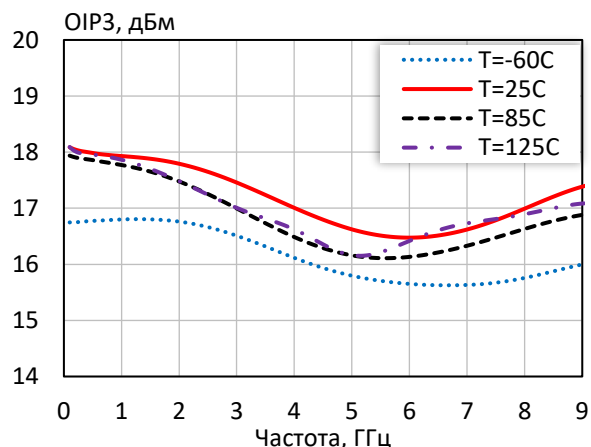
Точка пересечения интермодуляции третьего порядка по выходу при различной температуре ( I_p = 30\text{ mA} )
