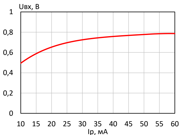
Выходное напряжение покоя U_{\text{вх}} при изменении режимного тока I_p
