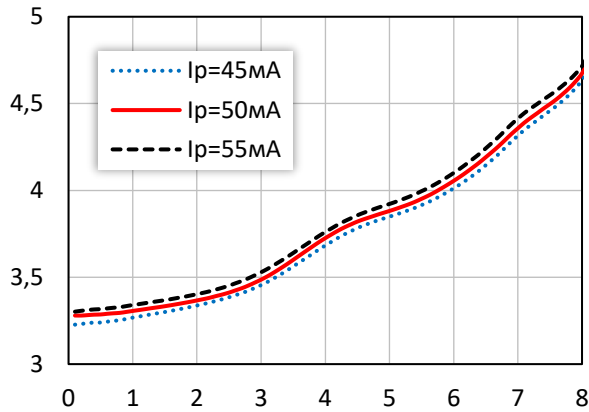
Коэффициент шума при различных режимных токах
