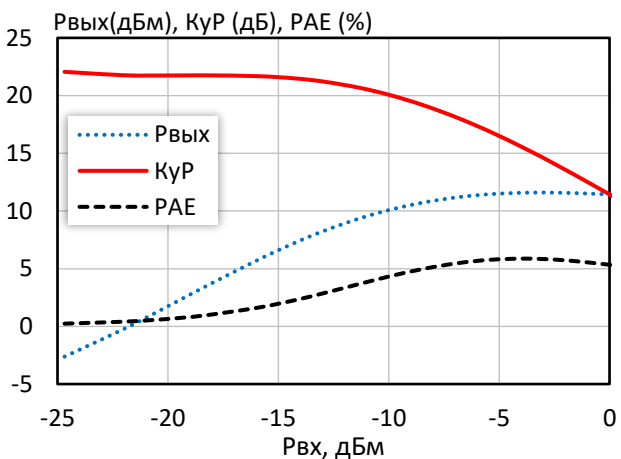
Выходная мощность, коэффициент усиления, КПД по добавленной мощности ( f = 3\text{ ГГц} , I_p = 50\text{ mA} )
