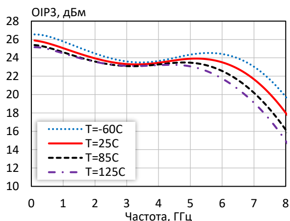
Точка пересечения интермодуляции третьего порядка по выходу при различной температуре ( I_p = 50\text{mA} )
