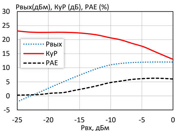
Выходная мощность, коэффициент усиления, КПД по добавленной мощности ( f = 10\text{ МГц} , I_p = 50\text{ мА} )
