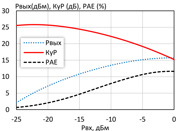
Выходная мощность, коэффициент усиления, КПД по добавленной мощности ( f = 3\text{ ГГц} , I_p = 50\text{ мА} )
