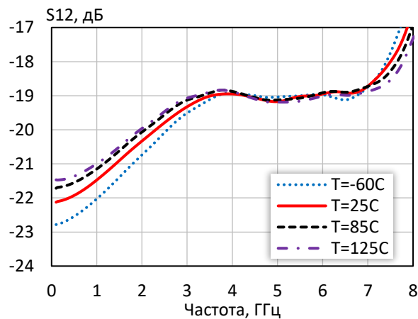
Коэффициент обратной передачи при различной температуре ( I_p = 30 мА)
