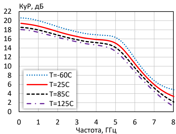
Коэффициент усиления при различной температуре ( I_p = 30 мА)
