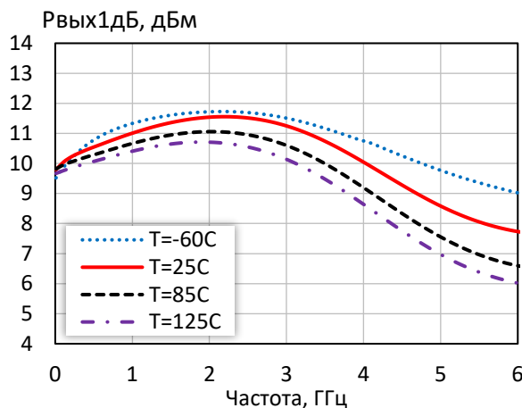
Выходная мощность при уровне компрессии КуР на 1 дБ при различной температуре ( I_p = 30\text{mA} )
