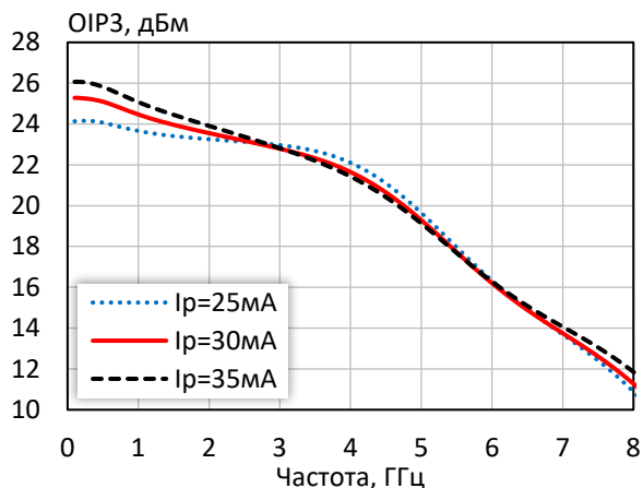
Точка пересечения интермодуляции третьего порядка по выходу при различных режимных токах
