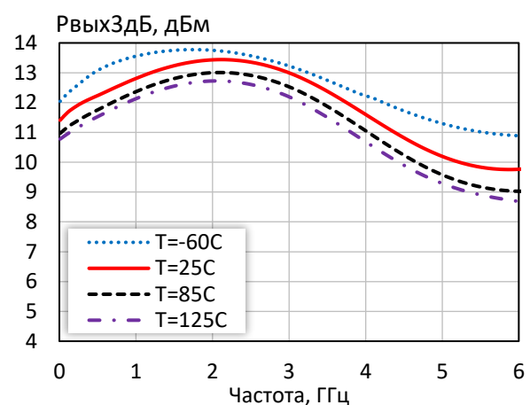
Выходная мощность при уровне компрессии КуР на 3 дБ при различной температуре ( I_p = 30\text{mA} )
