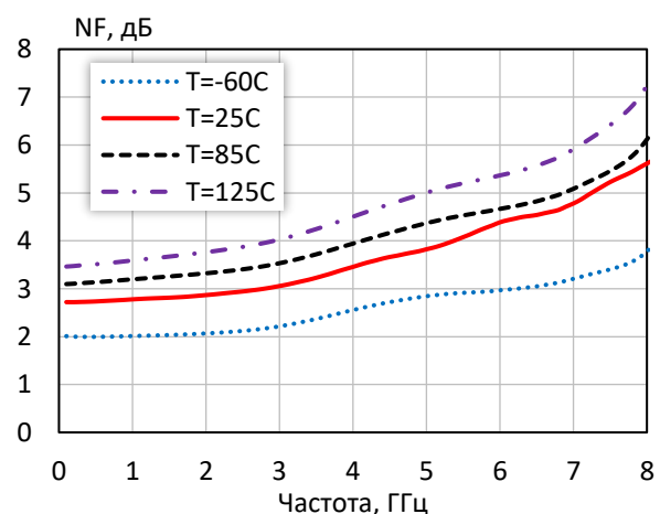
Коэффициент шума при различной температуре ( I_p = 30\text{mA} )
