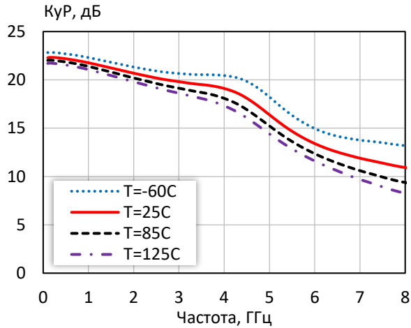
Коэффициент усиления при различной температуре ( I_p = 30 мА)
