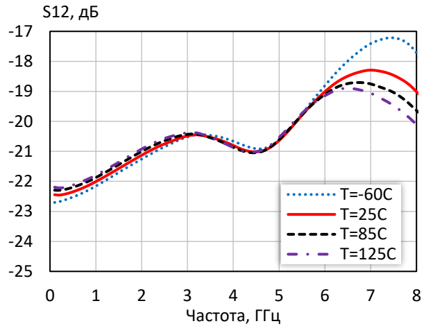
Кoeffициент обратной передачи при различной температуре ( I_p = 50 мА)
