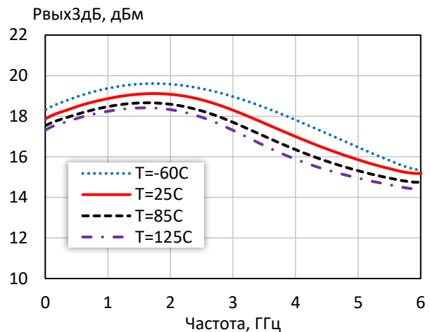
Выходная мощность при уровне компрессии K_{ур} на 3 дБ при различной температуре ( I_p = 50 мА)
