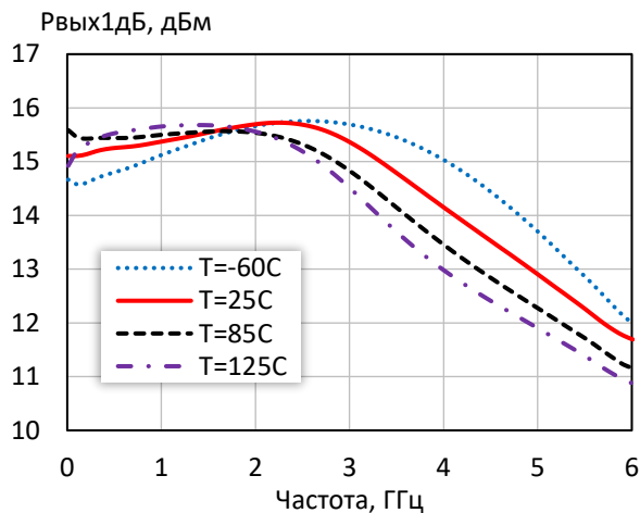
Выходная мощность при уровне компрессии K_{ур} на 1 дБ при различной температуре ( I_p = 50 мА)
