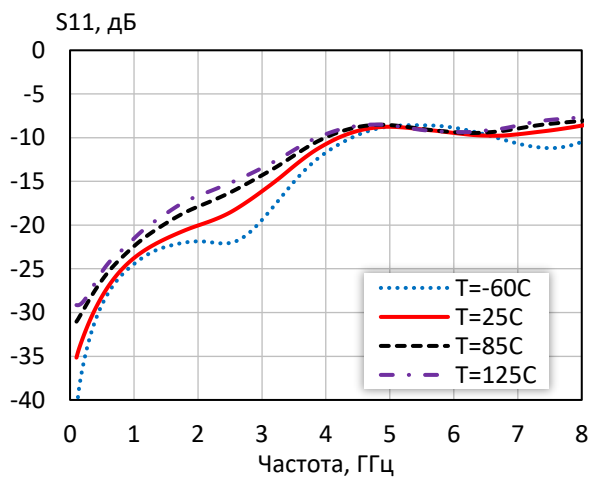
Кoeffициент отражения от входа при различной температуре ( I_p = 50 мА)
