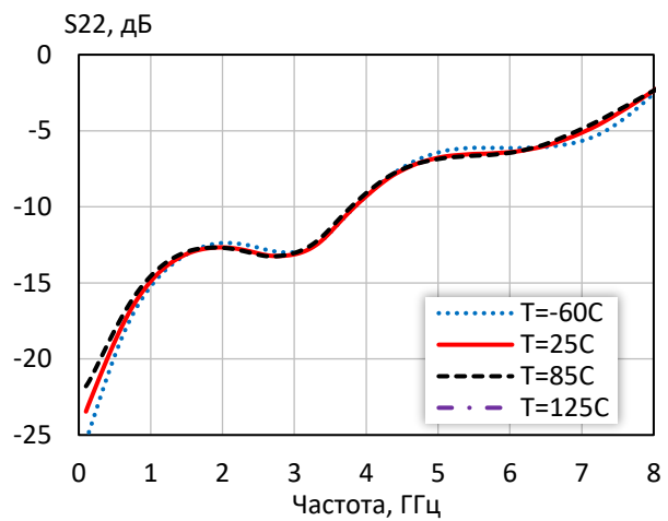
Кoeffициент отражения от выхода при различной температуре ( I_p = 50 мА)
