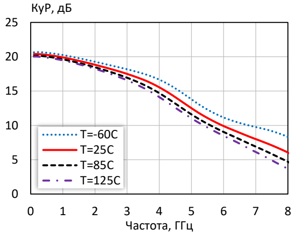
Кoeffициент усиления при различной температуре ( I_p = 50 мА)
