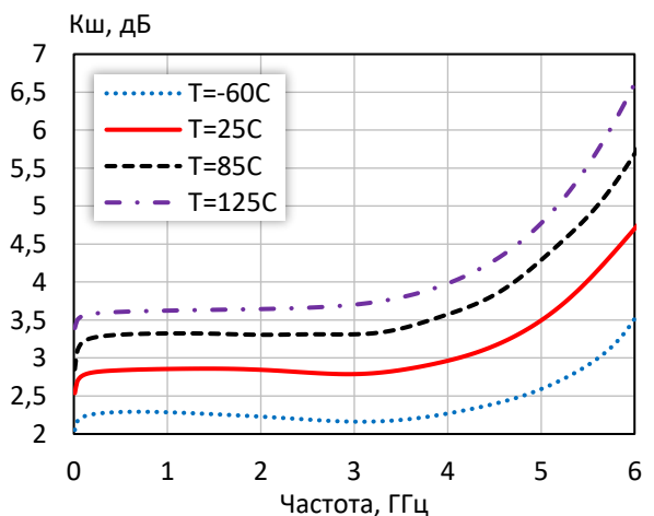
Коэффициент шума при различной температуре (Ip = 30 мА)
