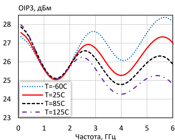
Точка пересечения интермодуляции третьего порядка по выходу при различной температуре
